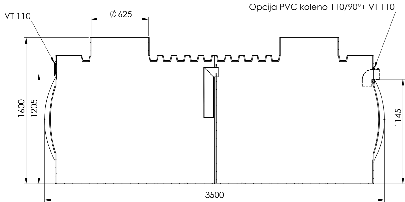
SECTION B-B SCALE 1 : 20
