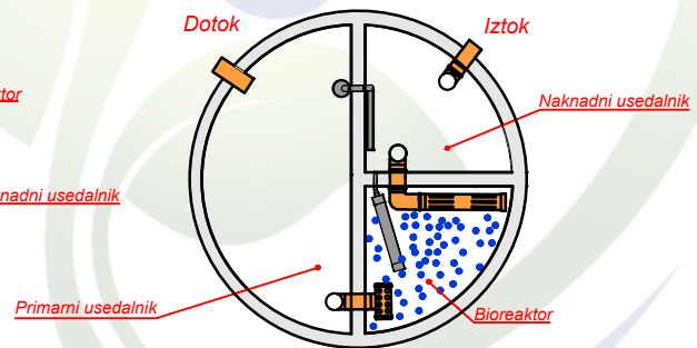
Možnost postavitve iztoka v levo stran
